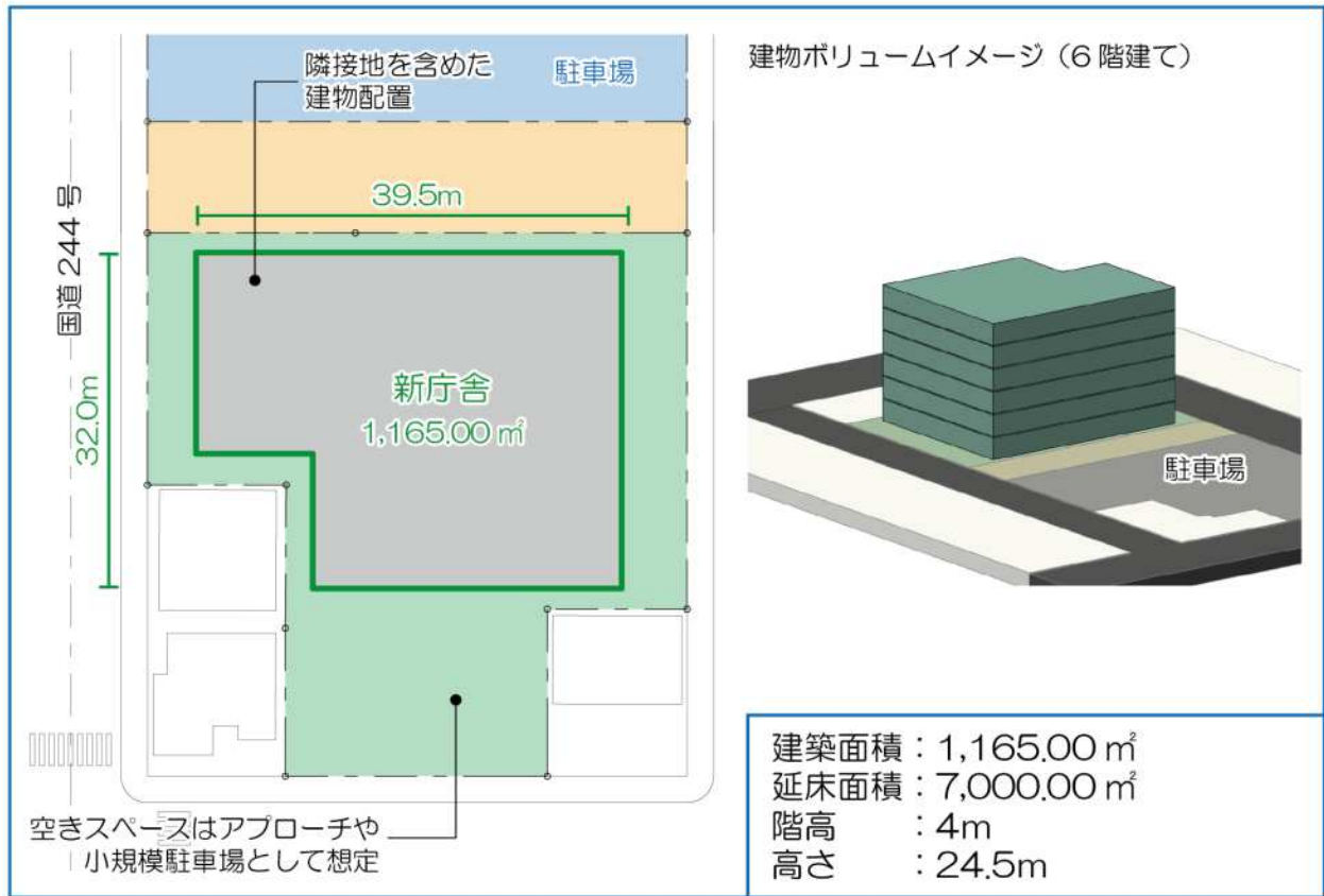
<表：建物ボリューム（建築・延床面積、階、高さ）のイメージ>
